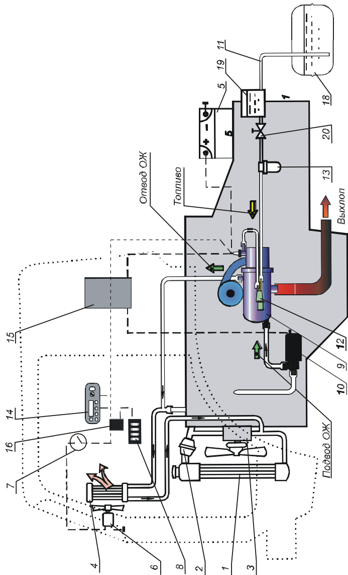
Рисунок 3 - Схема подключения подогревателя 1 - радиатор системы охлаждения автомобиля; 2 - термостат охлаждающей жидкости; 3 - автомобильный водяной насос; 4 - теплообменник системы отопления; 5 - аккумуляторная батарея; 6 - вентилятор системы отопления; 7 - выключатель вентилятора; 8 - блок предохранителей; 9 - подогреватель; 10 - электродвигатель с насосом; 11 - топливopровод; 12 - электромагнитный топливный насос; 13 - топливный фильтр; 14 - таймер-терморегулятор; 15 - блок управления работой подогревателя; 16 - реле управления работой вентилятора системы отопления; 18 - топливный бак автомобиля; 19 - бак топливный; 20 - кран питания подогревателя топливом.
